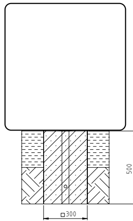
Polygoon ingebed in beton door middel van de vloerankers.
