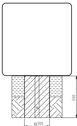
Cilinder ingebed in beton door middel van de vloeranker.
